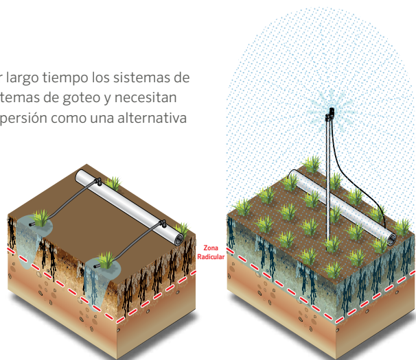
Espaciamiento del emisor 0,61 m (2 pies) Espaciamiento de línea de goteo 0,61 m (2 pies)
